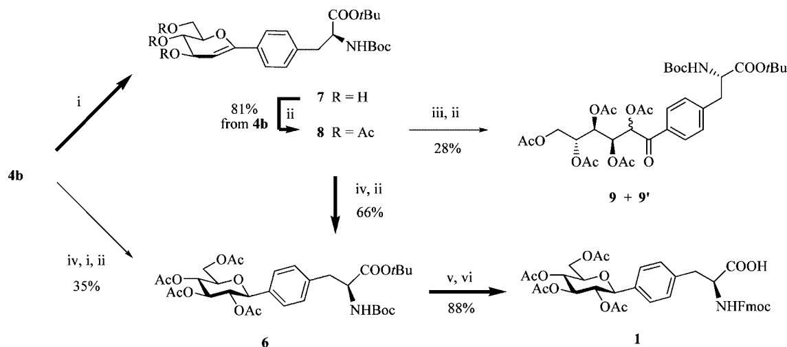
Scheme 4. Reagents and conditions: i) n\text{Bu}_4\text{NF} , THF, 0 °C to room temp.; ii) \text{Ac}_2\text{O} , pyridine, DMAP, room temp.; iii) \text{OsO}_4 , NMO, THF, t\text{BuOH} , pyridine, \text{H}_2\text{O} ; iv) \text{BH}_3\cdot\text{THF} , then \text{NaOH} , \text{H}_2\text{O}_2 ; v) TFA, \text{CH}_2\text{Cl}_2 ; vi) FmocOSu, \text{NEt}_3 , \text{CH}_3\text{CN}/\text{H}_2\text{O} .
